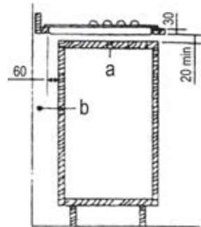
a՝ շարժուն պանել b՝ տարածությունը միացման համար
