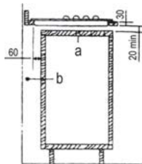
a – пересувна панель b – простір для з'єднання
