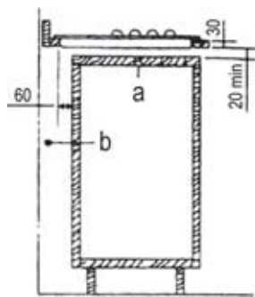
a – передвижная панель b – пространство для соединения
