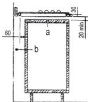
a – жылжытылатын тақта b – жалғауға арналған кеңістік
